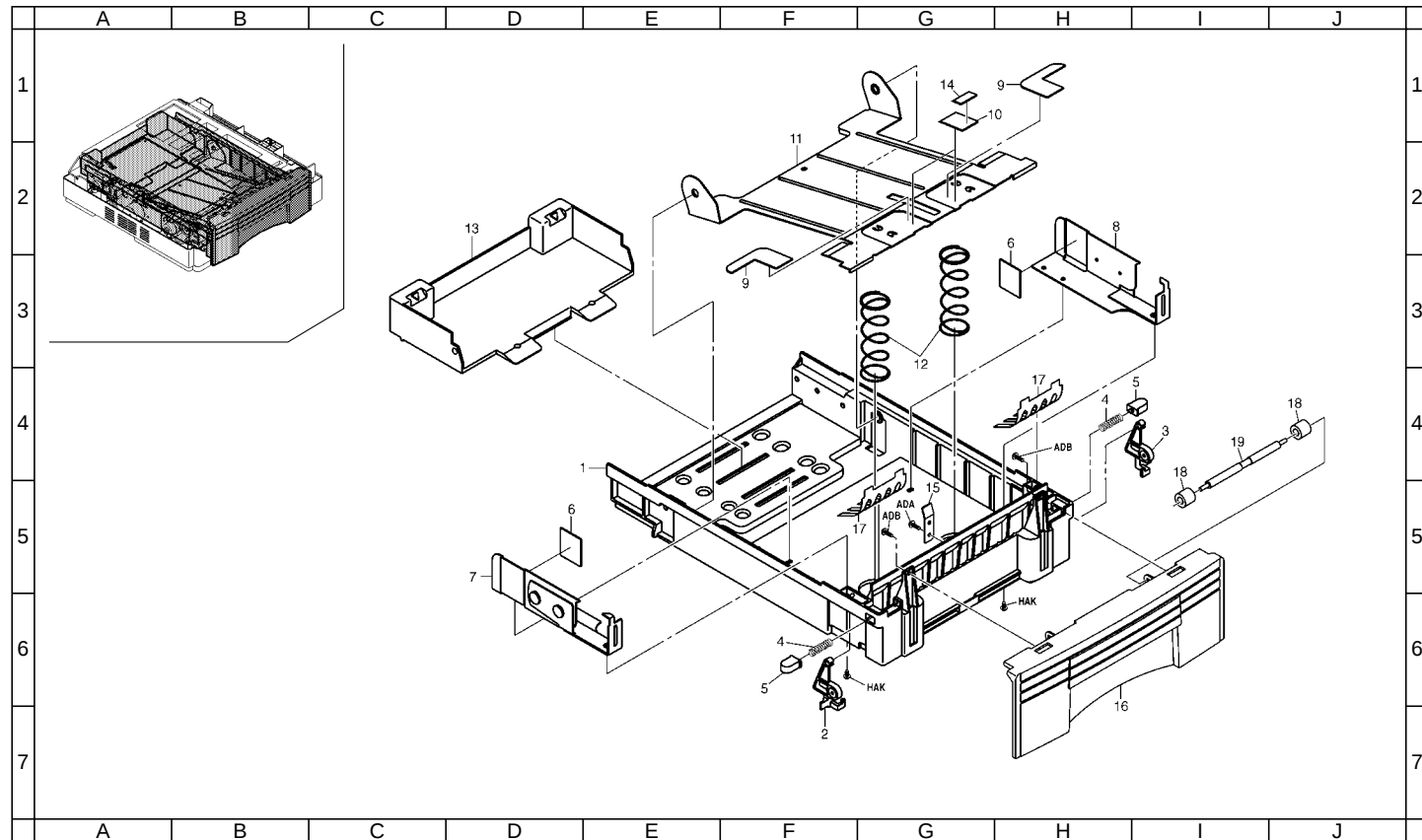
FIG. 2 CASSETTE
